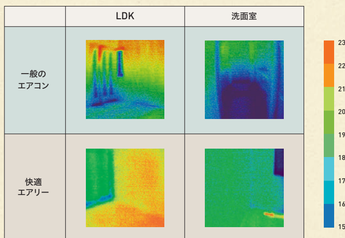
LDK・洗面室の上下温度の実測結果(1階)
