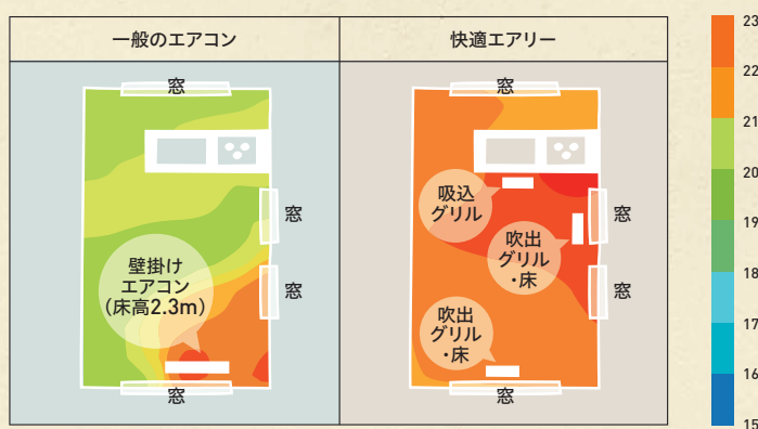
LDKの水平温度シミュレーション(1階)
